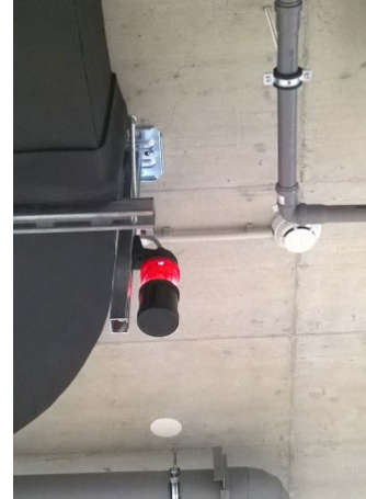
Slika 24: Svetlobni in zvočni signal detekcije tehničnega plina
