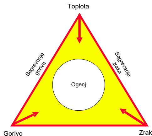
Slika 19: Požarni trikotnik
