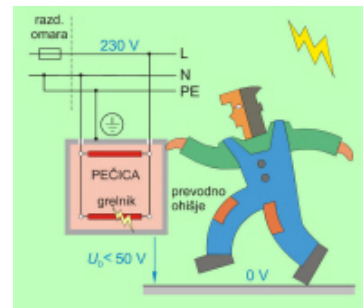
Slika 3: Posredni dotik
